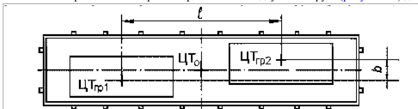
Рисунок 22 - Кососимметричное размещение грузов в вагоне
