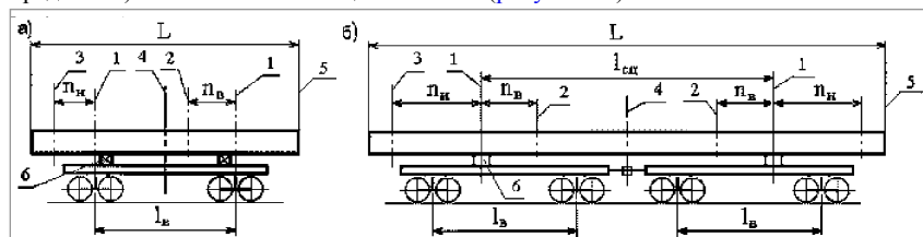
Рисунок 47 – Расчетные сечения длинномерного груза, размещенного а – на одиночном вагоне; б – на сцепе вагонов:
