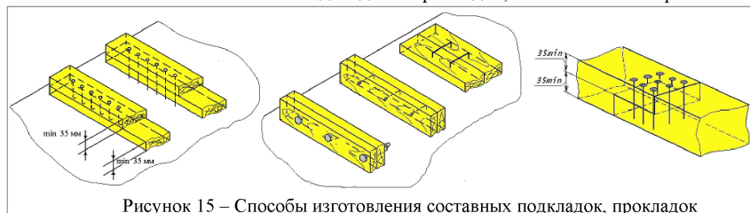
Рисунок 15 – Способы изготовления составных подкладок, прокладок
