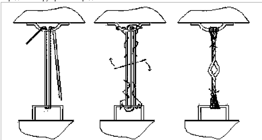
Рисунок 9 – Установка растяжек, обвязок по способу 3
