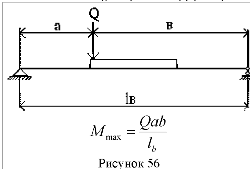
Схемы нагружения рамы вагона и формулы для расчета максимального изгибающего момента M_{max}
