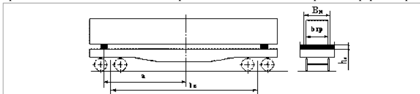
Рисунок 24 - Размещение груза на двух подкладках за пределами базы платформы
