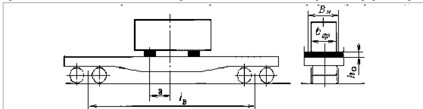
Рисунок 23 - Размещение груза на двух подкладках в пределах базы платформы
