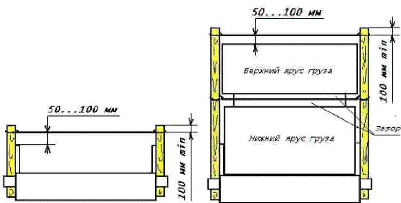
Рисунок 18 – Скрепление стоек на платформе
