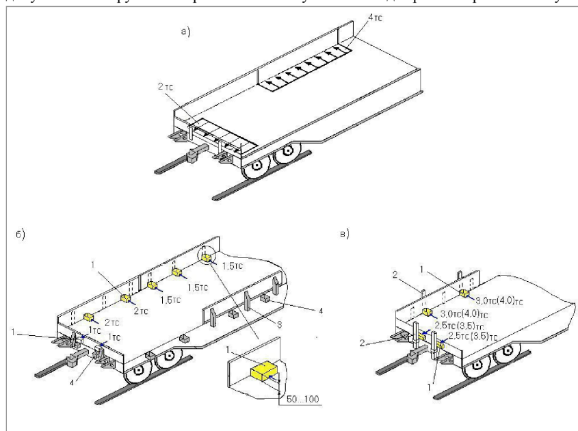
Рисунок 38- Схемы нагружения бортов платформ
