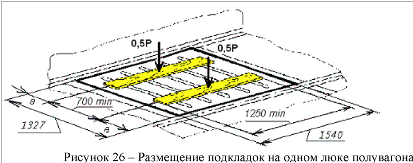
Рисунок 26 – Размещение подкладок на одном люке полувагона
