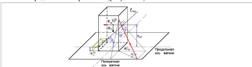
Рисунок 33-Углы наклона растяжки для крепления от опрокидывания груза в продольном направлении
