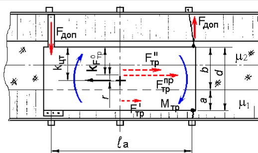
Рисунок 29-Схема для расчета дополнительного крепления груза от разворота
